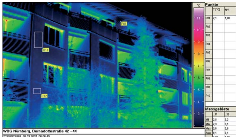
Infrarotthermografie der Südwestansicht
