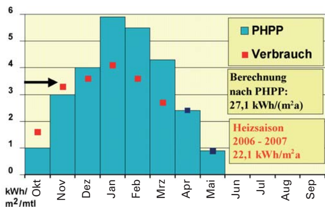
Abb. 1 Heizwärmebedarf gemäß PHPP-Berechnung und Messwerte für die Bestandswohnungen (Stand 1.4.2007)
