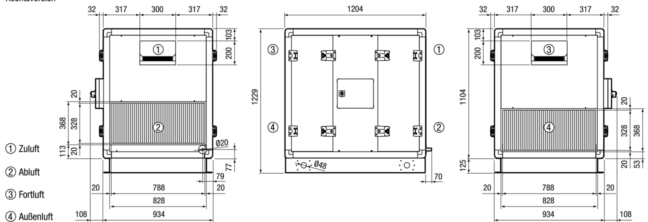
Reco-Boxx 1200 ZX-R Rechtsversion
