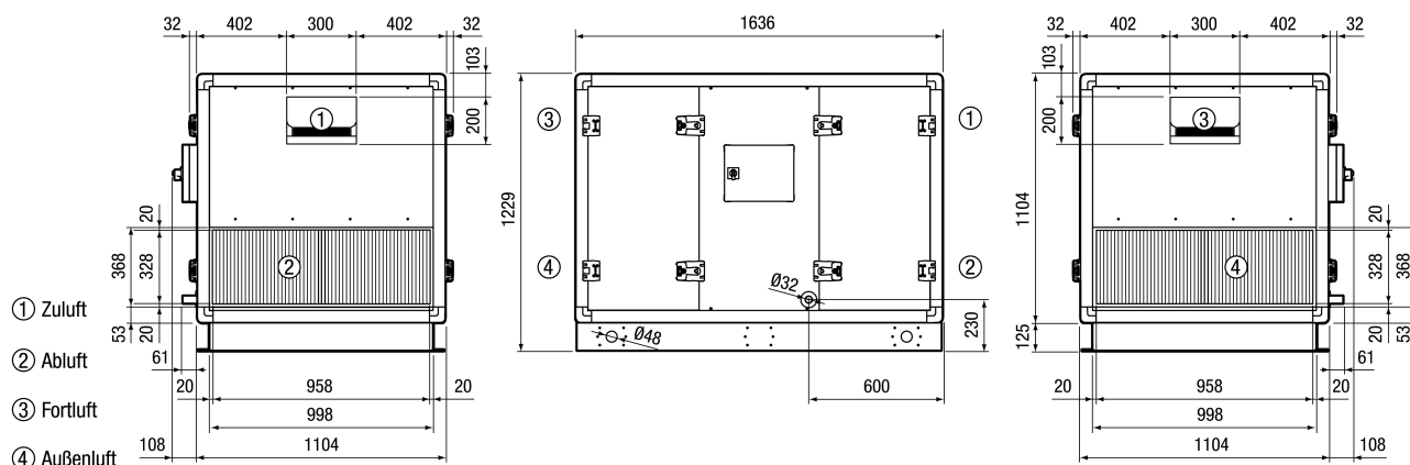
Reco-Boxx 2000 ZX-R Rechtsversion
