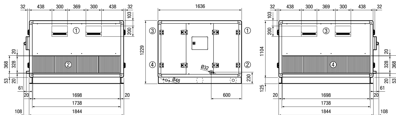
Reco-Boxx 4000 ZX-R Rechtsversion
