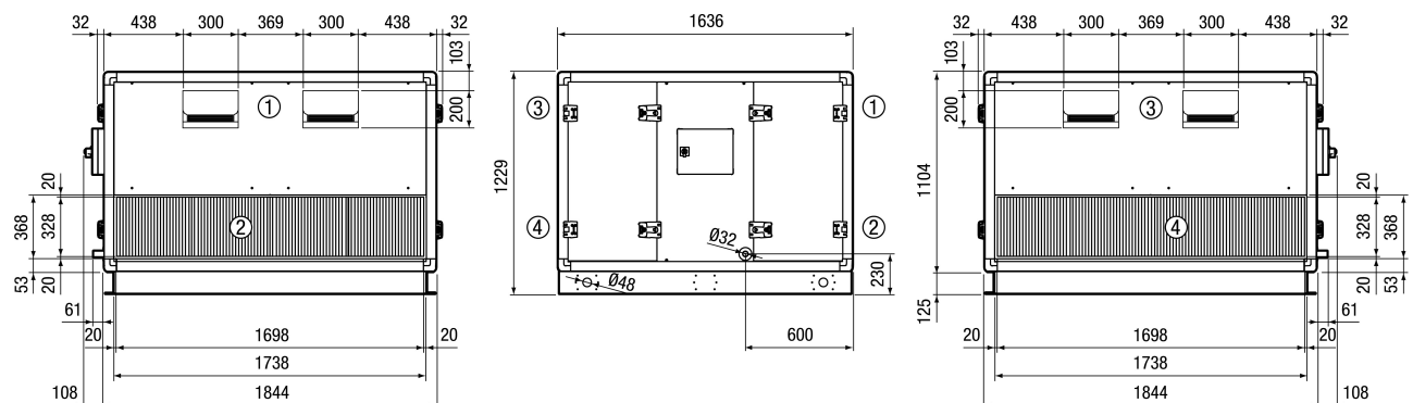
Reco-Boxx 4000 ZX-R Rechtsversion
