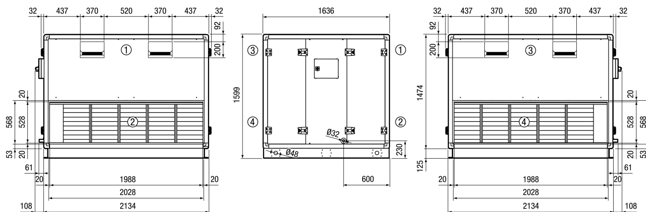
Reco-Boxx 6000 ZX-R Rechtsversion
