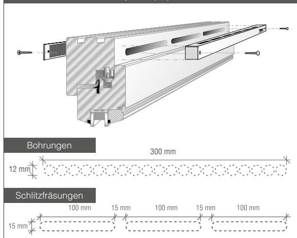
Einbau in Vollprofile (VP) wie Holzfenster
