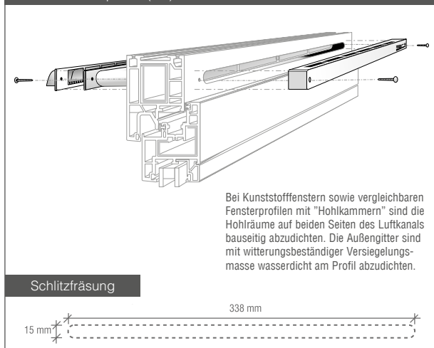
Einbau in Hohlprofile (HP) wie Kunststofffenster mit Luftkanal Fresh 33
