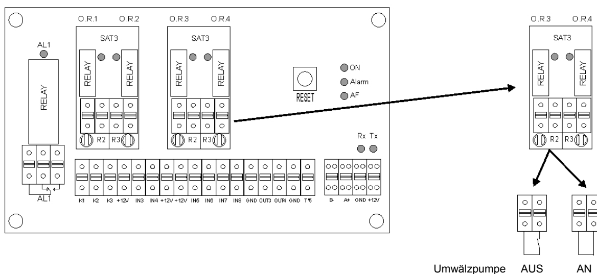
i/o Modul
