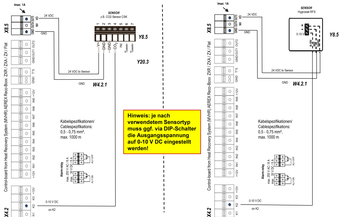
Anschlussplan Nr. 4.1
