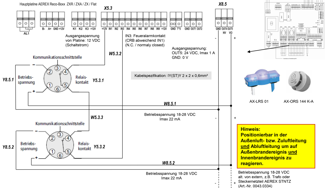
Anschluss 2 Lüftungsrauchscharter
