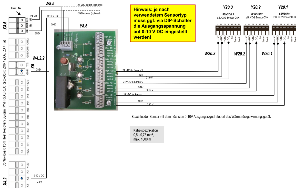
Anschlussplan Nr. 4.2
