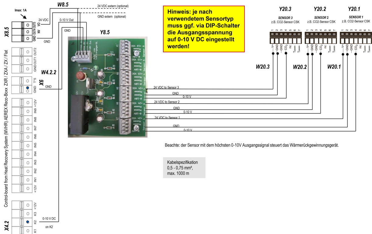
Anschlussplan Nr. 4.2
