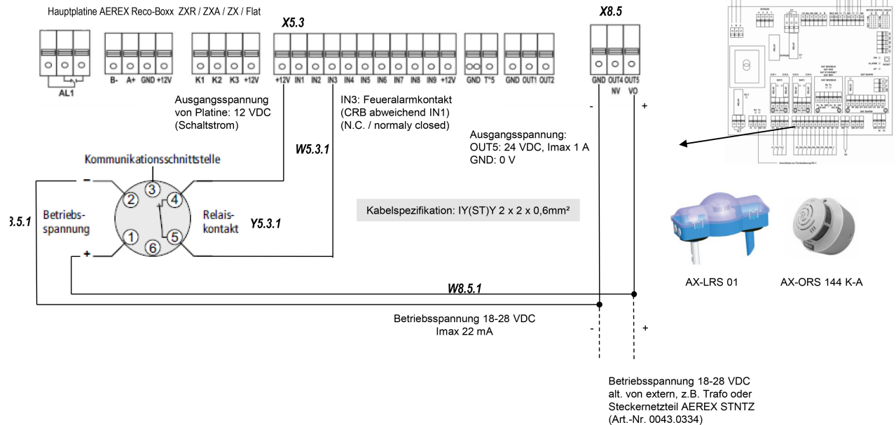
Anschlussplan Nr. 5
