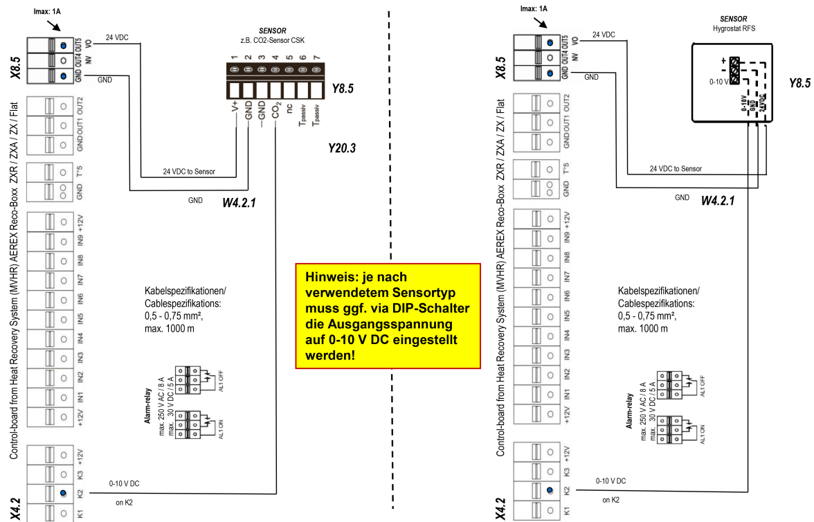
Anschlussplan Nr. 4.1
