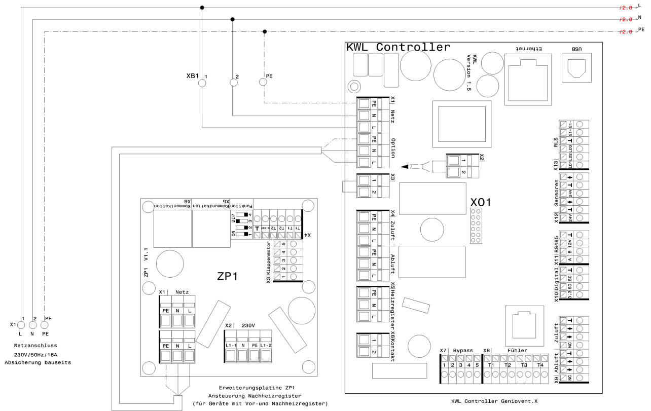
Schaltbild (Auszug). Die Gesamtübersicht Schaltbilder ist beim Produkt zu finden unter: Downloads / Planung / Schaltbilder Blatt 1: Platinenanschlussplan
