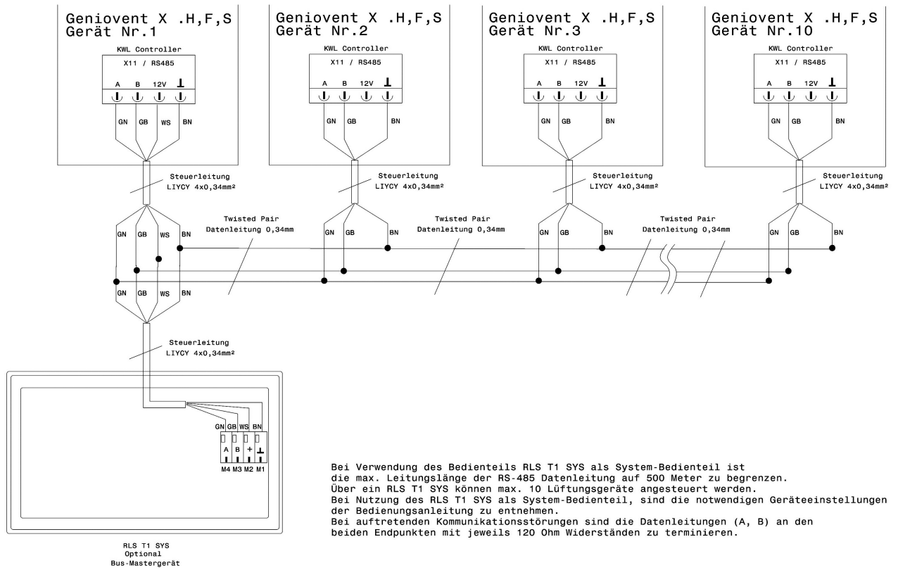
Schaltbild (Auszug). Die Gesamtübersicht Schaltbilder ist beim Produkt zu finden unter: Downloads / Planung / Schaltbilder Blatt 10: Anschlussbild Touchbedienteil RLS T1 SYS für Mehrgeräteanschluss (1 .... 10 Geräte)
